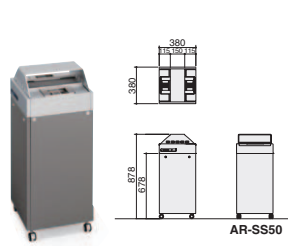
■エアリウムスタンド NEW!! (ロータイプ) AR-SS50 ¥312,900 (¥298,000) 外寸法/W380×D380×H878
