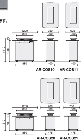
■エアリウムカウンター (壁面置きタイプ) AR-COS21swNN ¥619,500 (¥590,000) 外寸法/W1200×D750×H810
